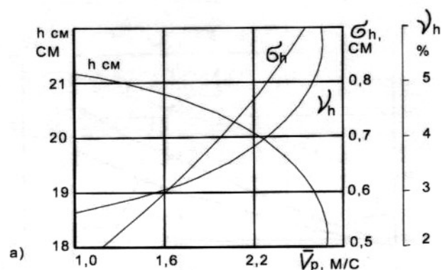
Рис. 7. Зависимости вероятностных оценок глубины обработки почвы h_{cm} от рабочей скорости движения МТА Т-4А+КМ-2,4
