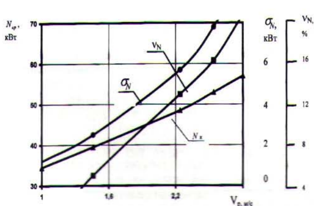
Рис.3. Зависимости вероятностных оценок тяговой мощности трактора Т-4А от скорости движения МТА Т-4А+КМ-2,4
