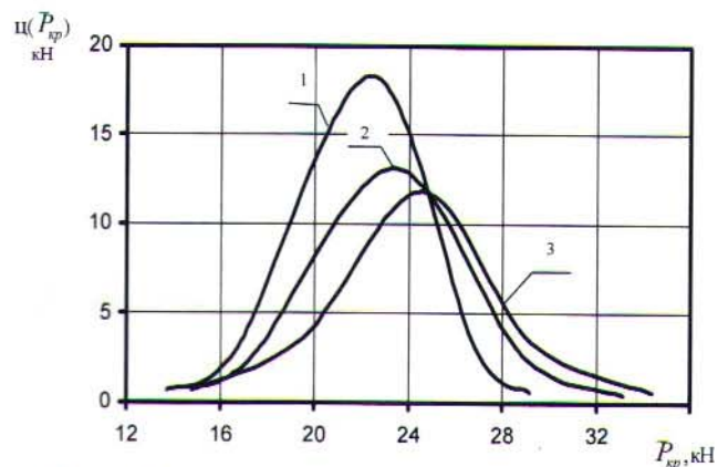
Рис.2. Плотности распределения вероятностей тягового усилия P_{кр} трактора МТА Т-4А+КМ-2,4: 1- V_p = 1,45 м/с; 2- V_p = 2,24 м/с; 3- V_p = 2,53 м/с.
