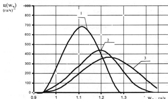
Рис. 6. Плотности распределения вероятностей часовой производительности МТА Т-4А+КМ-2,4: 1- \bar{V}_p=1,45 м/с; 2- \bar{V}_p=2,24 м/с; 3- \bar{V}_p=2,53 м/с.
