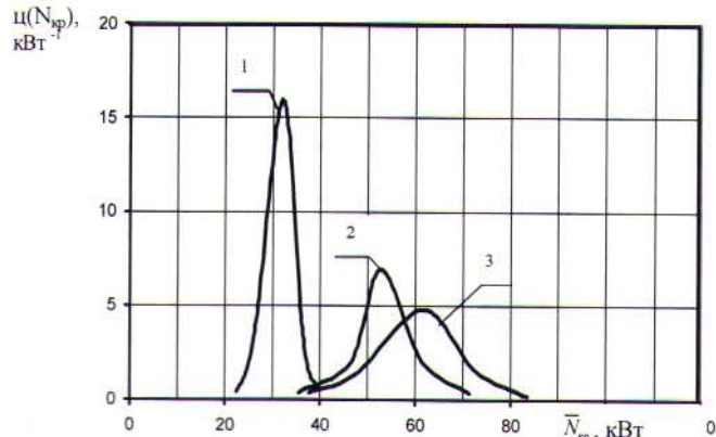
Рис.4. Плотности распределения вероятностей тяговой мощности N_{кр} трактора при работе МТА Т-4А+КМ-2,4: 1- \bar{V}_p = 1,45 м/с; 2- \bar{V}_p = 2,24 м/с; 3- \bar{V}_p = 2,53 м/с.
