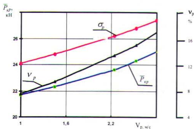
Рис.1. Зависимости вероятностных оценок тягового усилия P_{кр} трактора МТА Т-4А+КМ-2,4.
