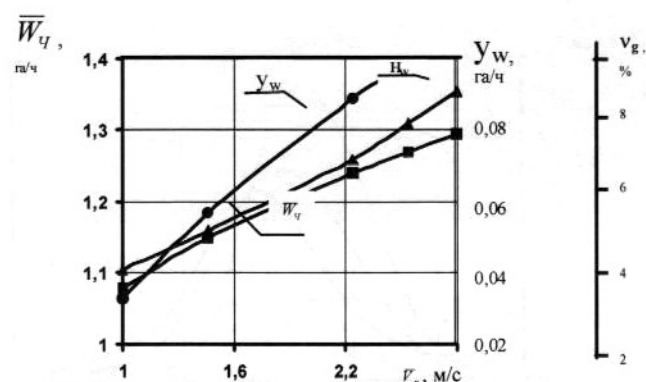
Рис. 5. Зависимости вероятностных оценок производительности МТА Т-4А+КМ-2,4 от скорости его движения
